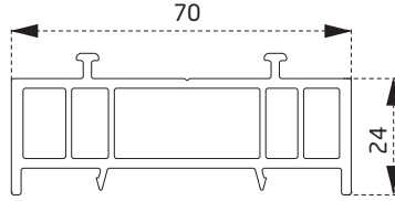
KZY06 Kasa Yükseltme Profili Frame Joint Profile
