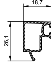
FA - 104 24mm.Cama Göre Çita Glazing Bead for 24mm Glass 0,263 kg/m
