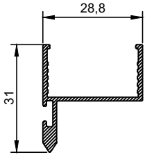
FS - 04 0,165 kg/mt Çift Cam Adaptörü Double Glass Adapter
