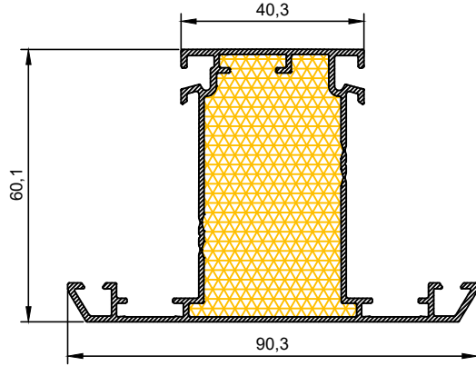
FA - 102 1,161 kg/mt Orta Kayıt Profili / Mullion Profile
